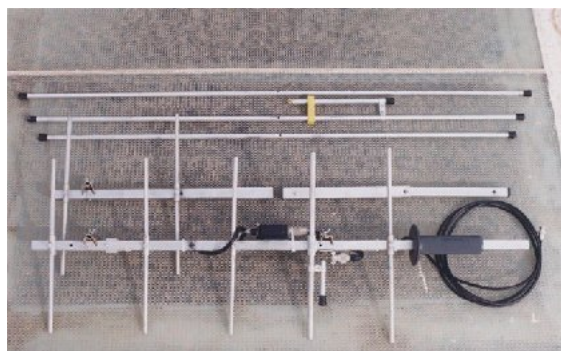
Foto 5: Antena desmontada para transporte
