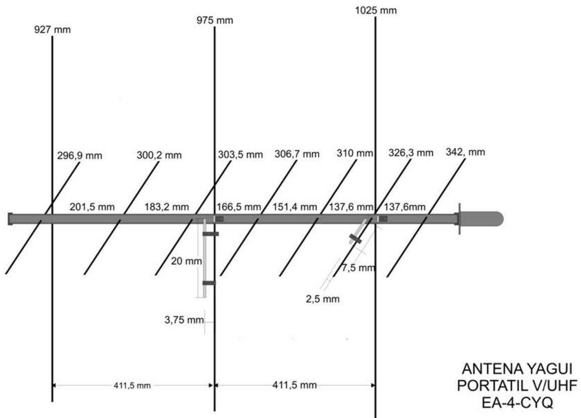
Figura n°1: Esquema de antena bibanda portable
